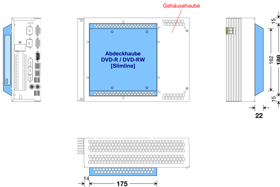
Abb. 5-1: Abdeckhaube für DVD-Laufwerk [Slimline]
